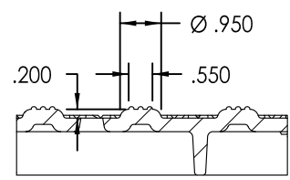
SECTION D-D SCALE 1 : 4
